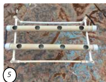
संरचना तैयार होने के बाद छिद्र वाले पाइप को स्टैंड पर स्थापित किया।
